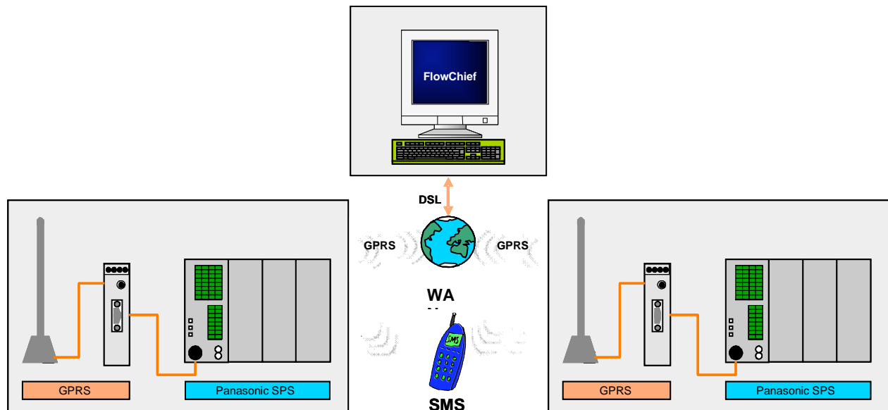
GPRS Kommunikation mit dem Prozessleitsystem FlowChief
